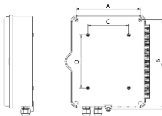
Рис. 2 Расположение отверстий для монтажа
