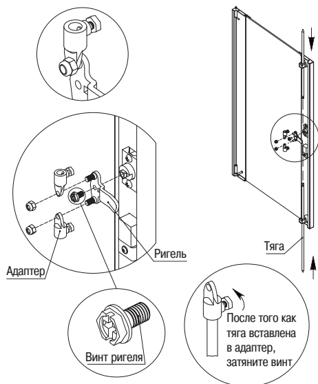
Рисунок 11 – Сборка дверей
