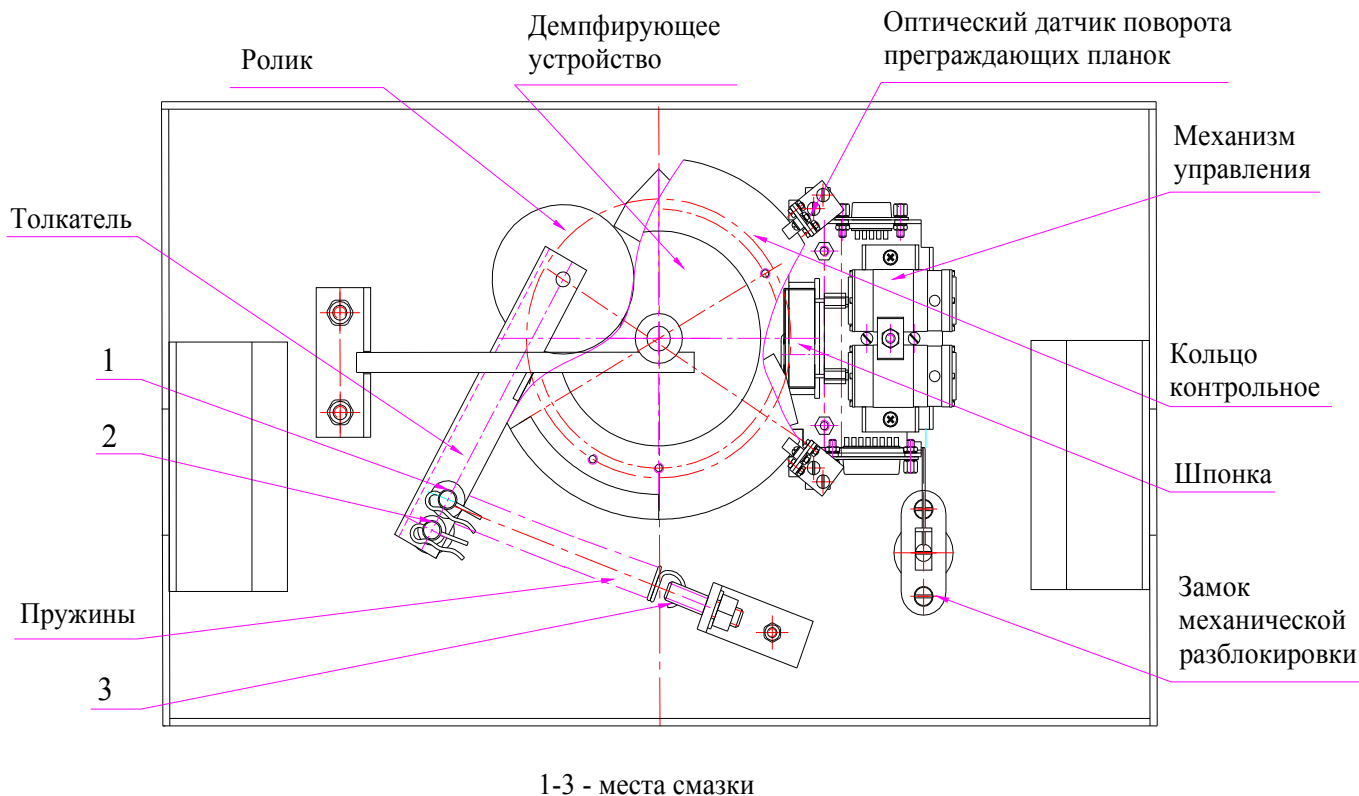
Рисунок 14 - Расположение внутренних деталей и узлов стойки турникета
