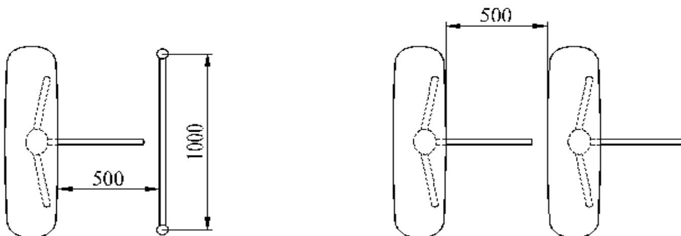
Рисунок 9 – Рекомендации по организации зоны прохода
