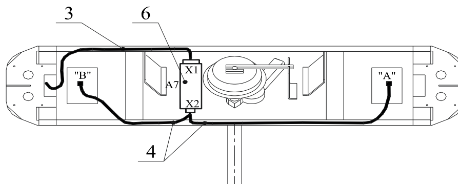
Рисунок 11 – Схема прокладки кабелей в стойке турникета:
