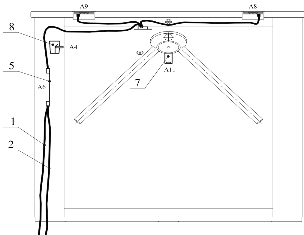
Вид со снятой крышкой
