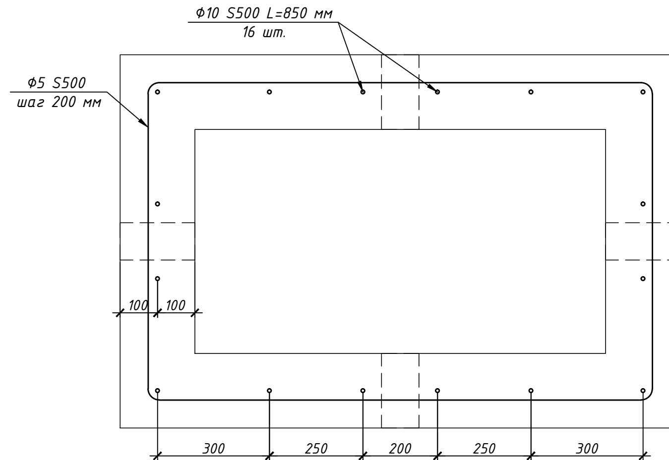
3-3 (армирование)
