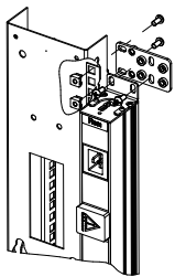
Установка блока розеток в стойки СТК
