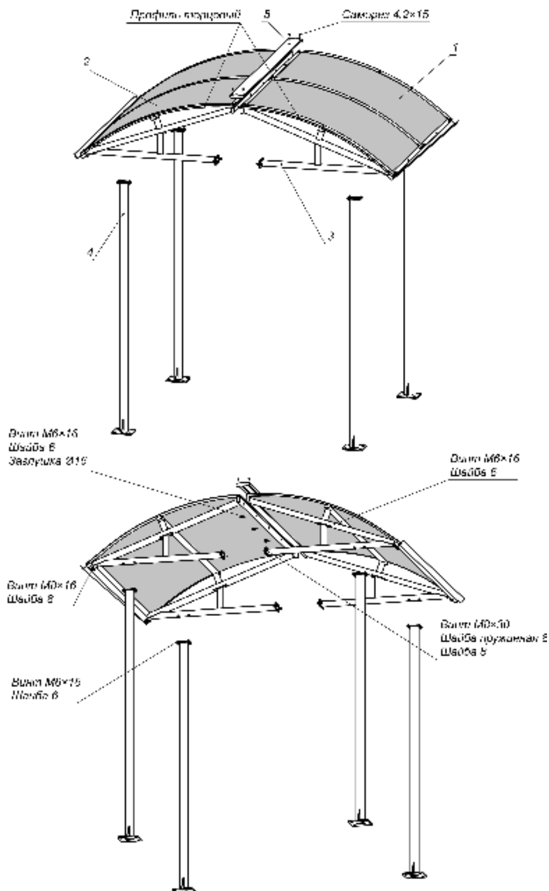
Рисунок 2. Устройство крыши:
