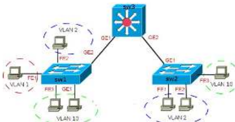
Рис. 5.3.14.1 Топология сети
