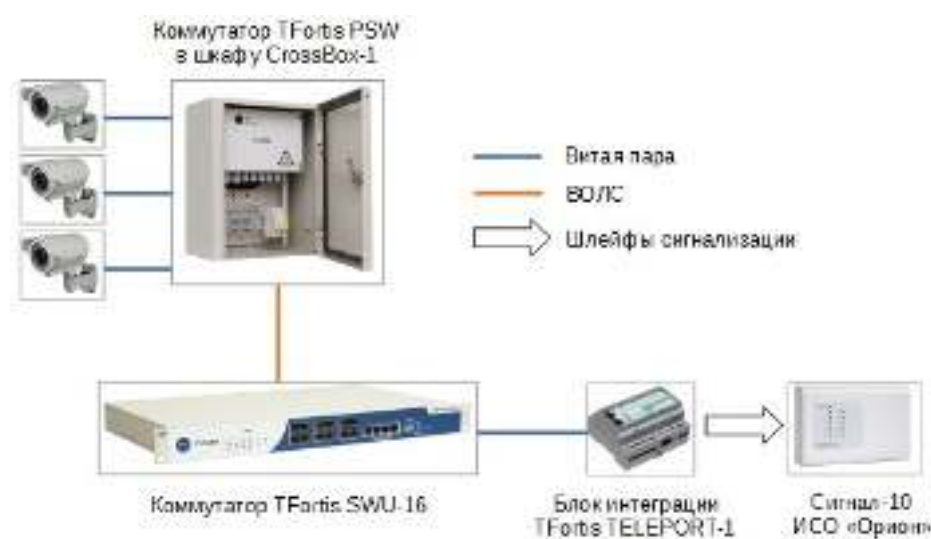
Рис. 5.3.27.1 Структура сети
