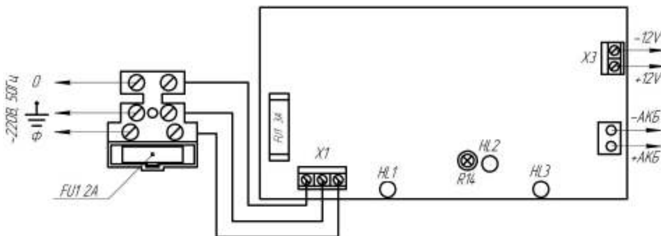
Рис. 1 Схема подключения
