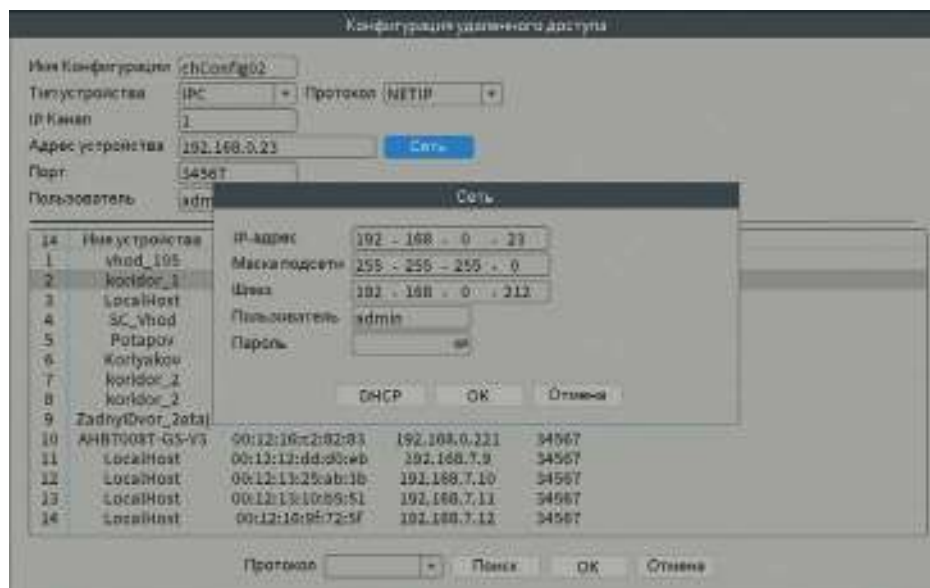
Рис.4.14 Интерфейс настройки IP адреса
