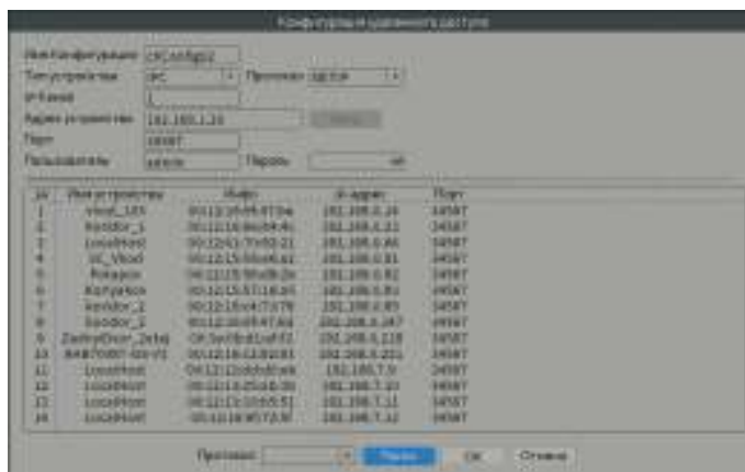
Рис.4.13 Интерфейс удаленной настройки канала
