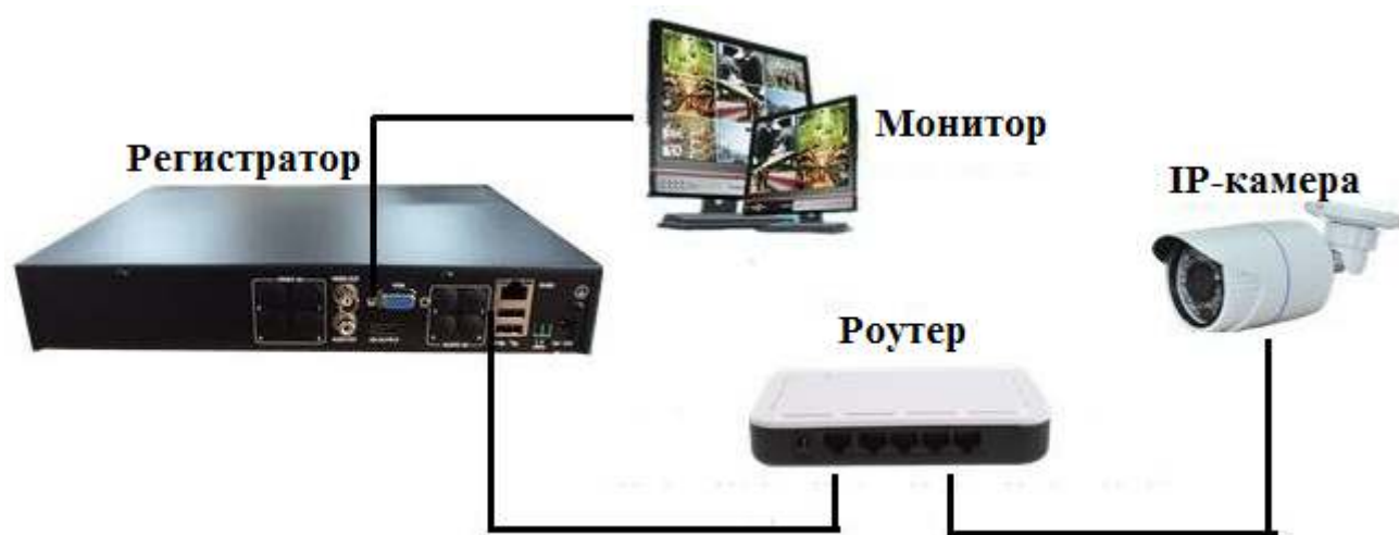
Рис. 2.1 Диаграмма подключения системы
