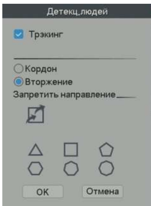
Рис.4.4 Настройка области обнаружения и трекинга
