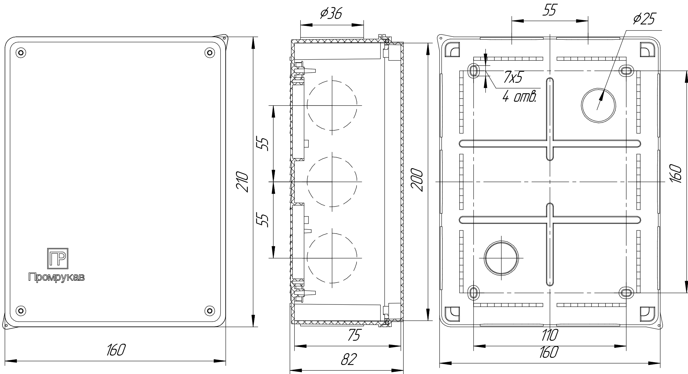
Коробка распределительная 40-03215 для о/п безгалогенная (HF) атмосферостойкая 200x150x75
