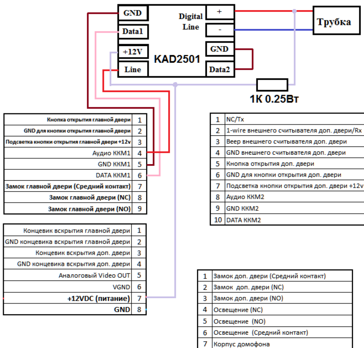
Схема подключения
