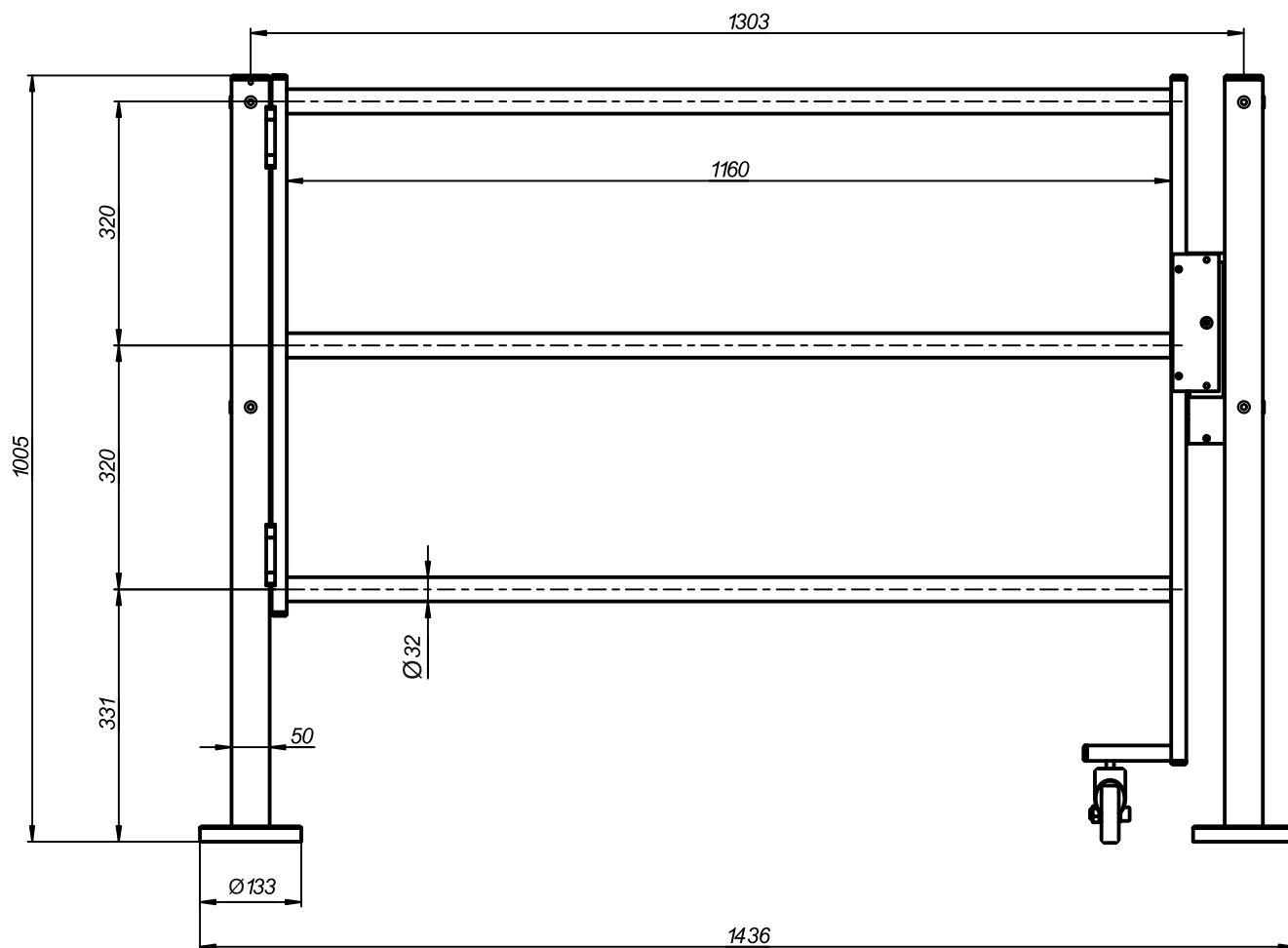
Рисунок 1. Габаритные размеры секции «Антипаника» с электромагнитным замком серии «RTA-02».
