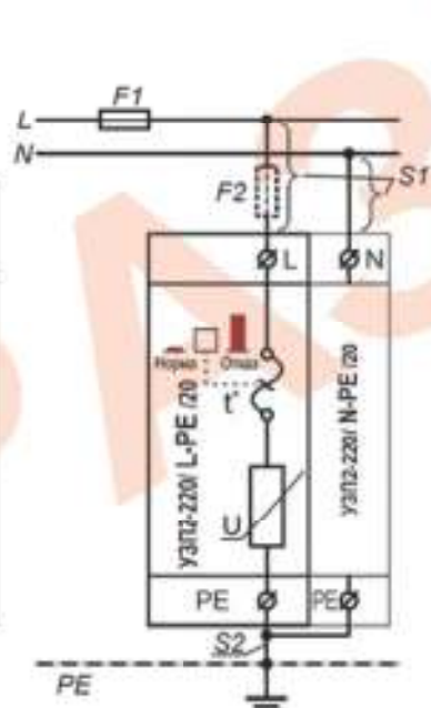
Рис.2 Схема подключения для однофазной сети
