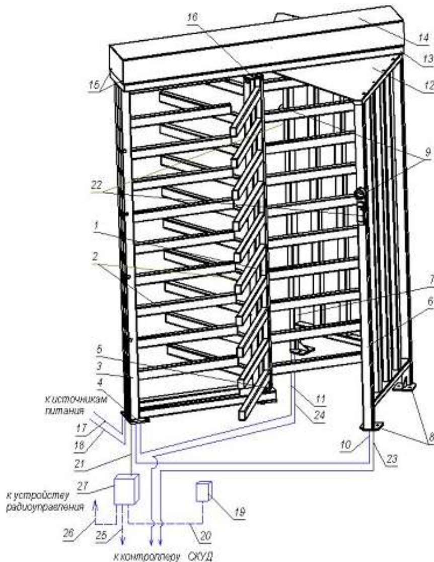
Рисунок 1 — Устройство турникета:
