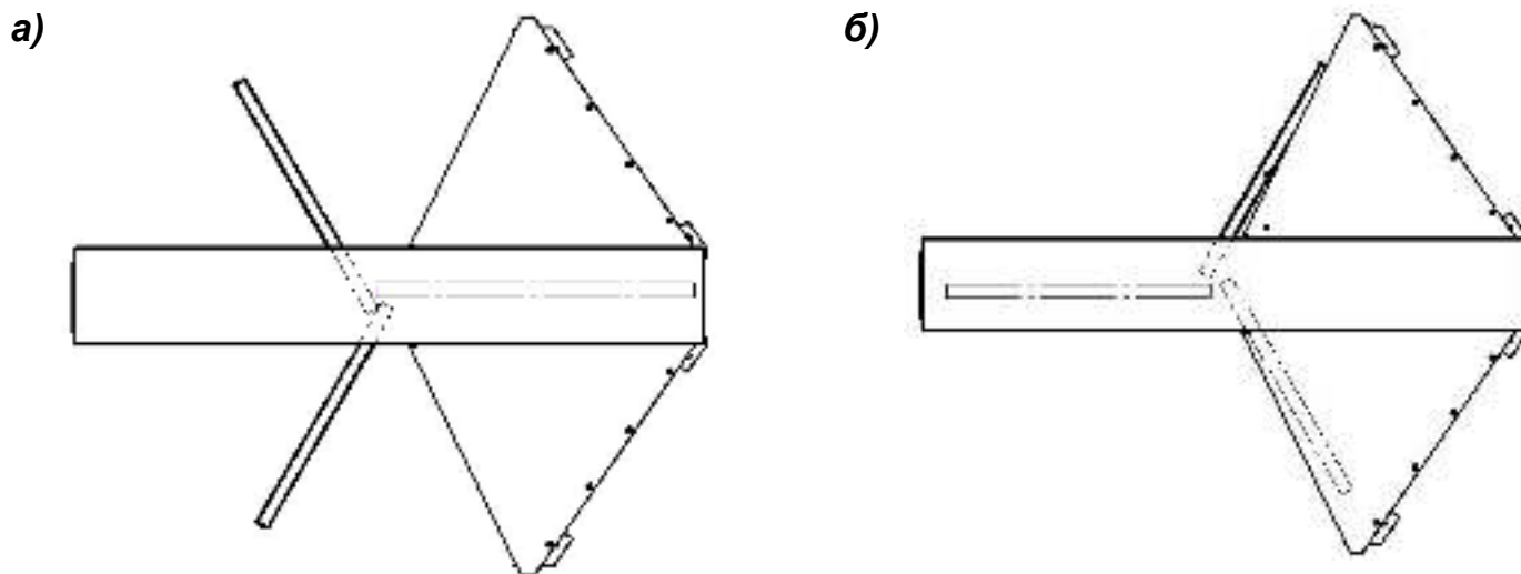
Рисунок 12 – Исходное положение створок турникета (вид сверху): а – для бесшлюзовых режимов работы; б – для шлюзовых режимов работы
