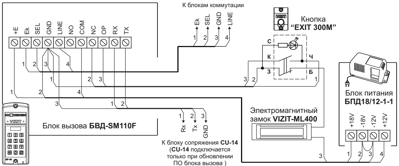
Рисунок 6 - Схема соединений блока вызова БВД-SM110F с электромагнитным замком VIZIT-ML400, блоком питания БПД18/12-1-1 и кнопкой "EXIT 300M"
