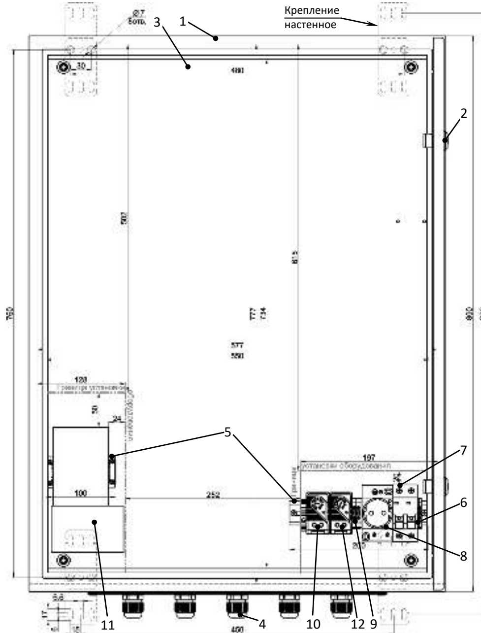
Рисунок 1 – Устройство шкафа
