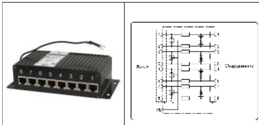
Рис.5 Внешний вид и электрическая схема SP-IP8/1000(ver.2)
