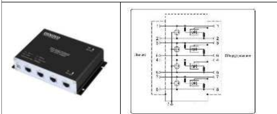
Рис.4 Внешний вид и электрическая схема SP-IP4/1000, SP-IP4/1000P
