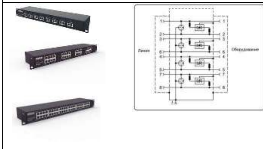
Рис.6 Внешний вид и электрическая схема SP-IP8/1000R, SP-IP8/1000PR, SP-IP16/1000R, SP-IP24/1000R, SP-IP16/1000PR, SP-IP24/1000PR
