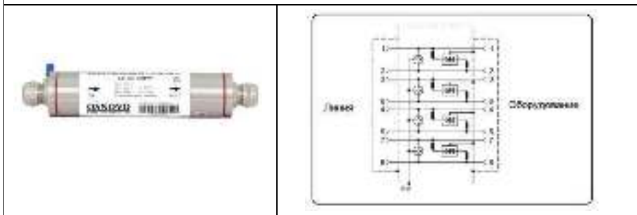
Рис.3 Внешний вид и электрическая схема SP-IP/1000PW
