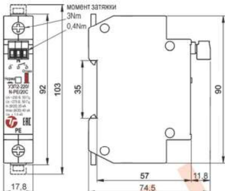
Рис.1 Габаритные размеры
