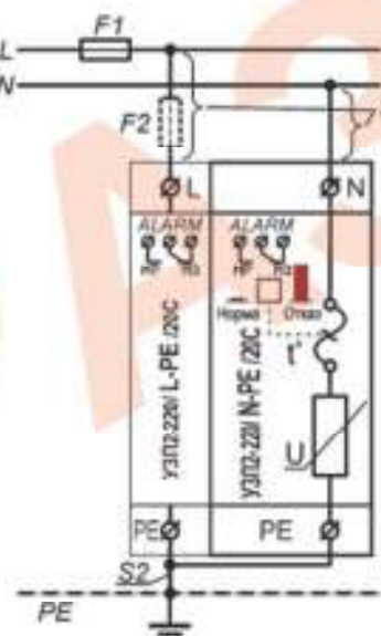
Рис.2 Схема подключения для однофазной сети
