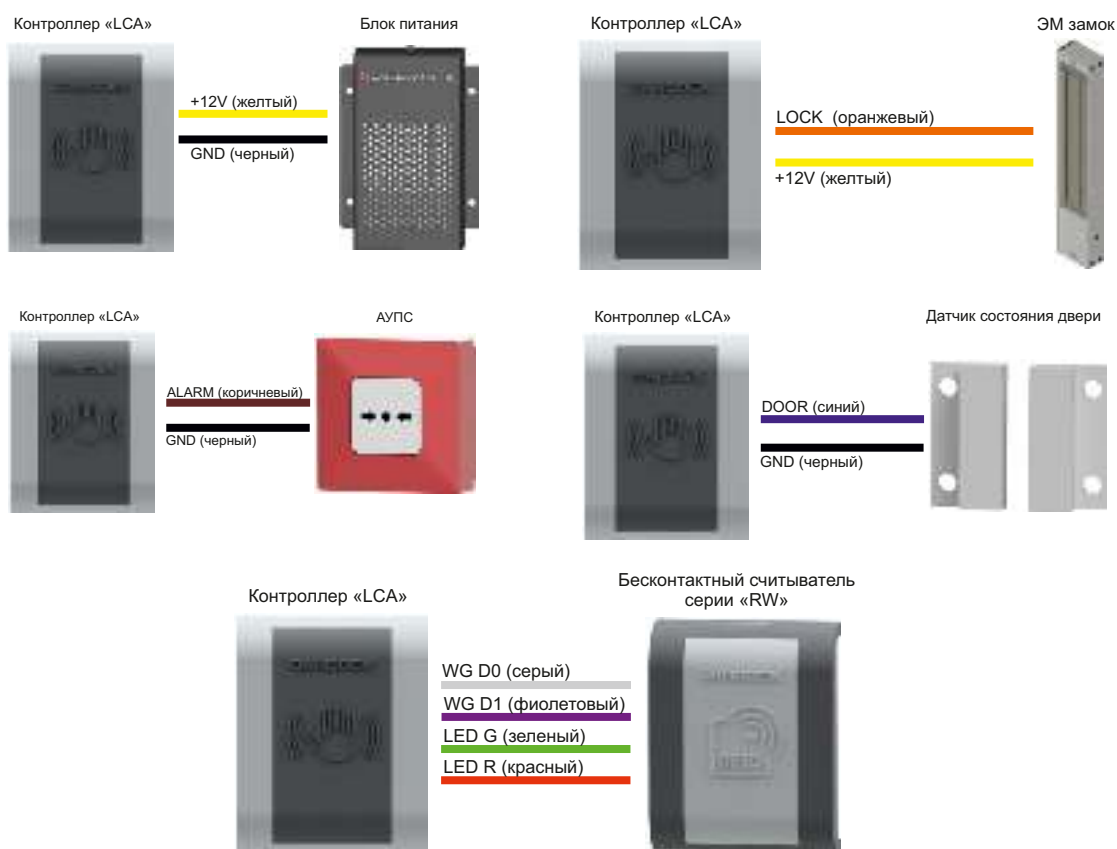
Рисунок 4.1 Подключение устройств к «LCA»
