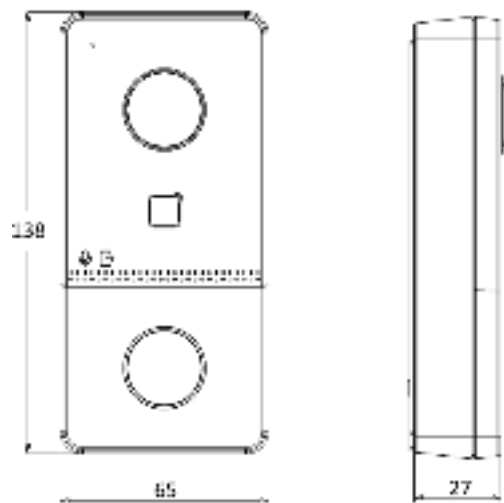
Вызывная панель
