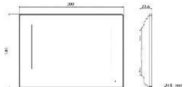
Экран видеодомофона
