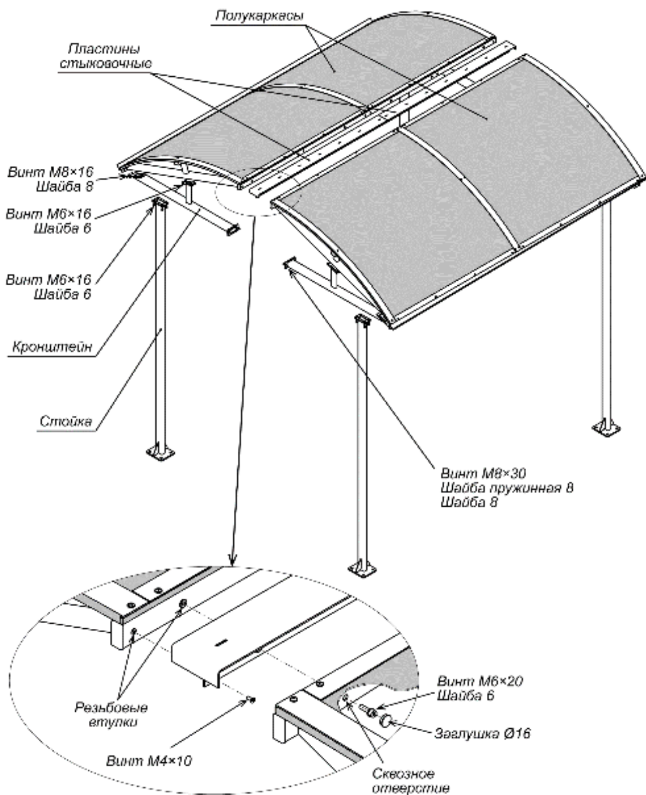
Рисунок 2. Устройство крыши
