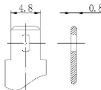
Позиция клемм
