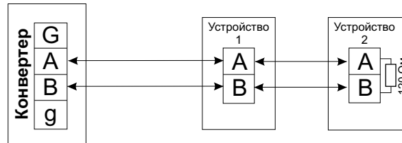
Схема подключения устройств с интерфейсом RS-485.
