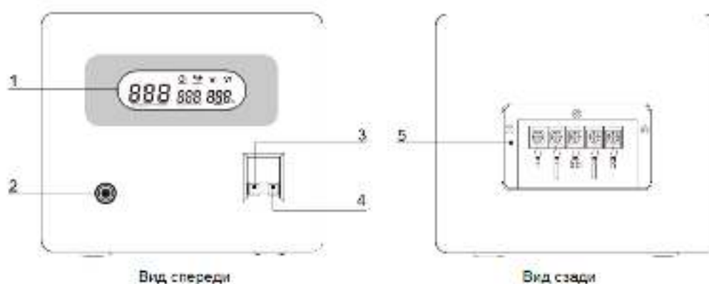
Рисунок 3. Внешний вид стабилизаторов напряжения SMARTWATT AVR TOWER 3000-5000VA. Описание элементов приводится в таблице 3.
