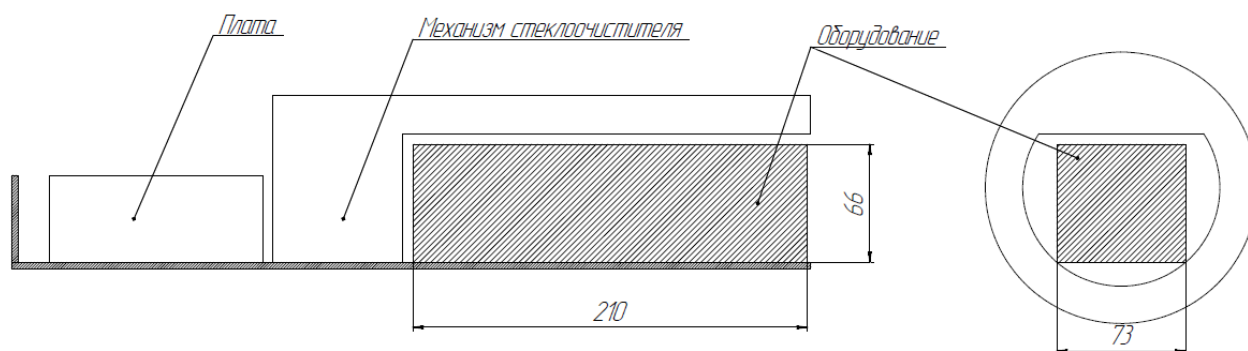
Рисунок А2 – Полезный объем термокожуха для установки видеооборудования – 73х66х210 (габариты видеооборудования, ШхВхГ, мм)
