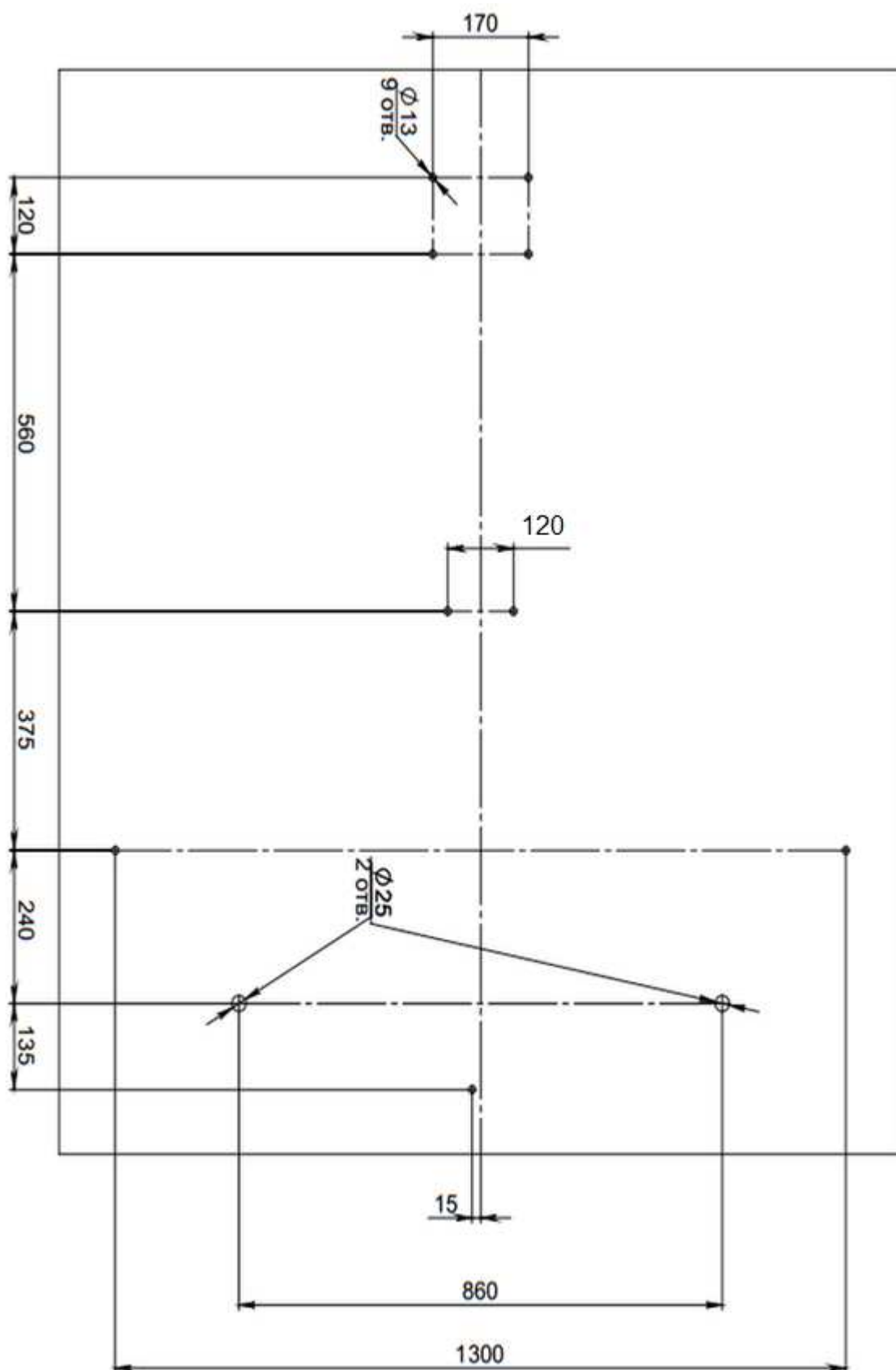
Рис. 21. Установочные размеры турникета
