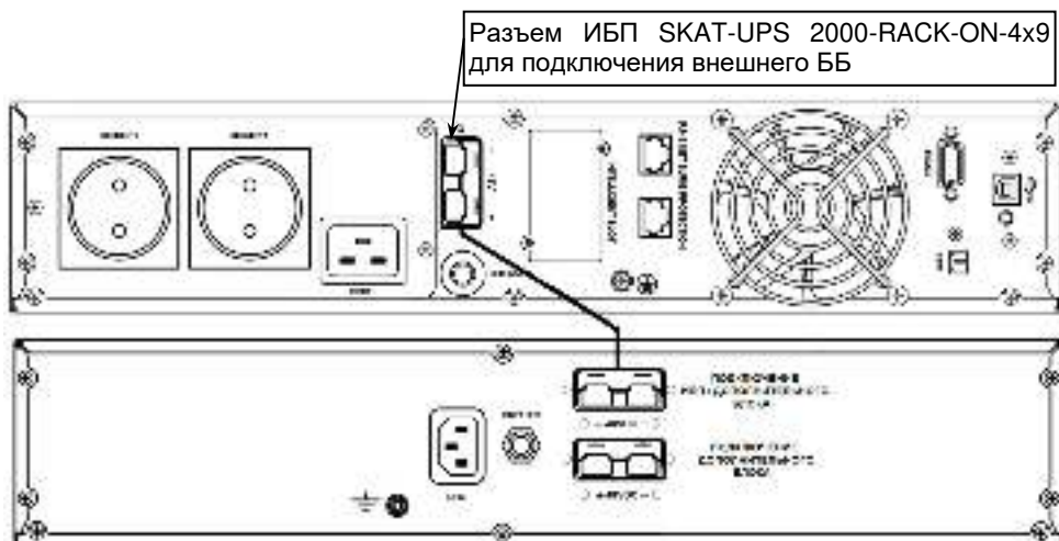
Рисунок 5 – Схемы подключения ББ к ИБП SKAT-UPS 2000-RACK-ON-4x9-E и SKAT-UPS 2000-RACK-ON-4x9
