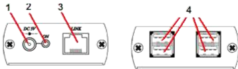
Рис. 4 Вид спереди и сзади UE03T
