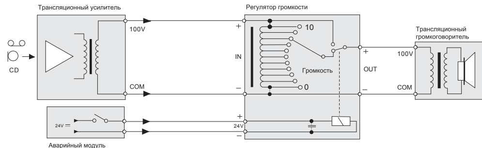
Схема подключения
