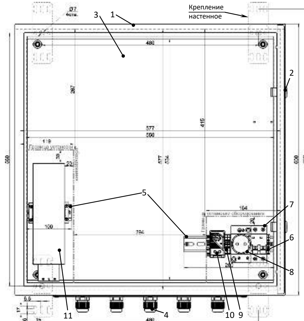
Рисунок 1 – Устройство шкафа
