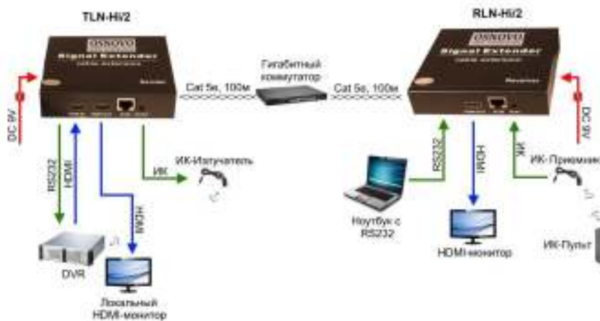
Рис. 5 Схема подключения комплекта TLN-Hi/2+RLN-Hi/2 в режиме «точка-точка» через гигабитный коммутатор
