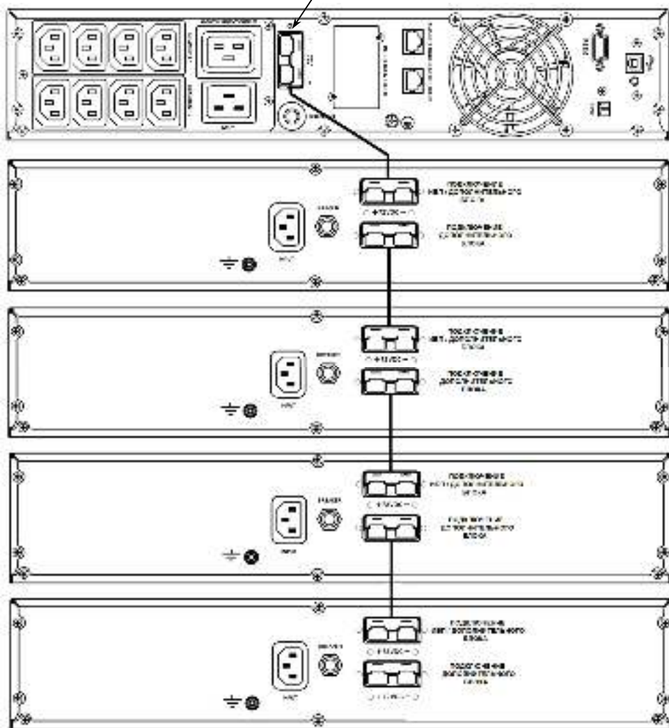
Рисунок 6 – Схема подключения нескольких ББ к ИБП (Продолжение на стр. 10)
