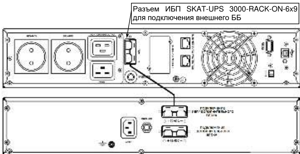
Рисунок 5 – Схемы подключения ББ к ИБП SKAT-UPS 3000-RACK-ON-6x9-E и SKAT-UPS 3000-RACK-ON-6x9
