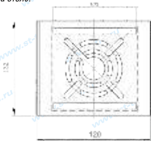
Рис.1 Габаритные размеры
