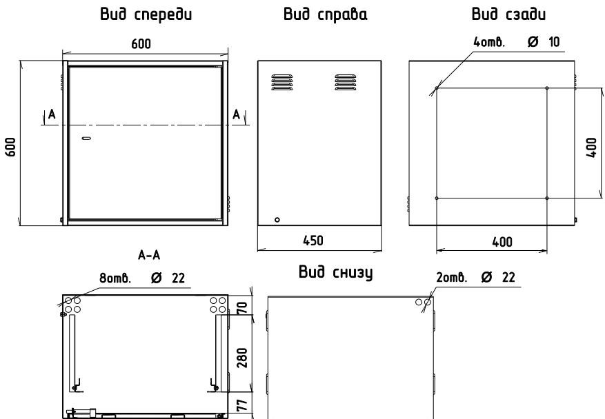
Чертеж шкафа
