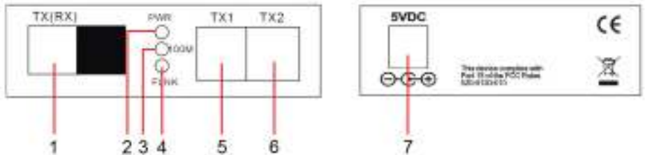
Рис. 5 Элементы медиаконвертеров OMC-100-21S5a (OMC-100-21S5b)
