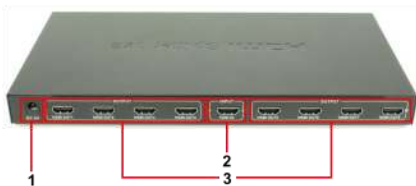
Рис.3 HDMI разветвитель D-Hi1081, разъемы и индикаторы на задней панели
