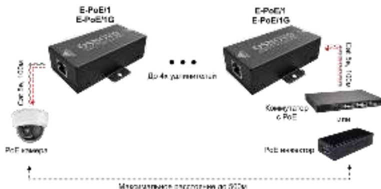
Рис. 7 Схема подключения удлинителей на примере модели E-PoE/1, E-PoE/1G
