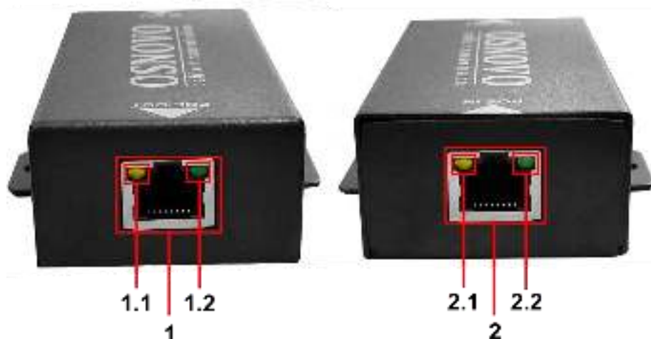
Рис. 3 Удлинители E-PoE/1, E-PoE/1G, разъемы и индикаторы
