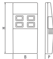
Габаритные размеры передатчиков (мм)
