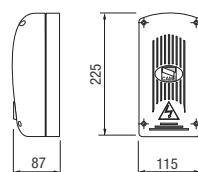
Габаритные размеры приемников (мм)
