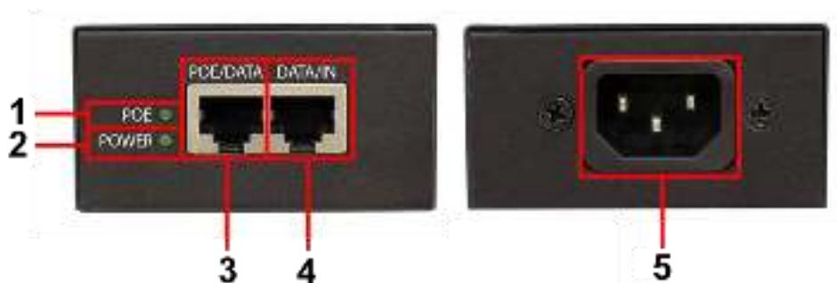
Рис. 2 Midspan-1/902G, разъемы на передней и задней панелях
