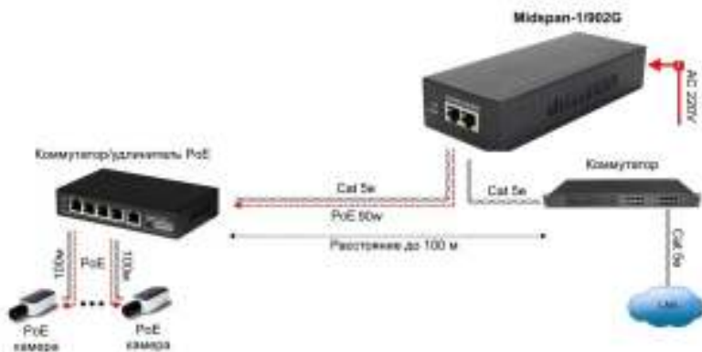
Рис.4 Типовая схема подключения инжектора Midspan-1/902G вместе с PoE коммутатором/удлинителем
