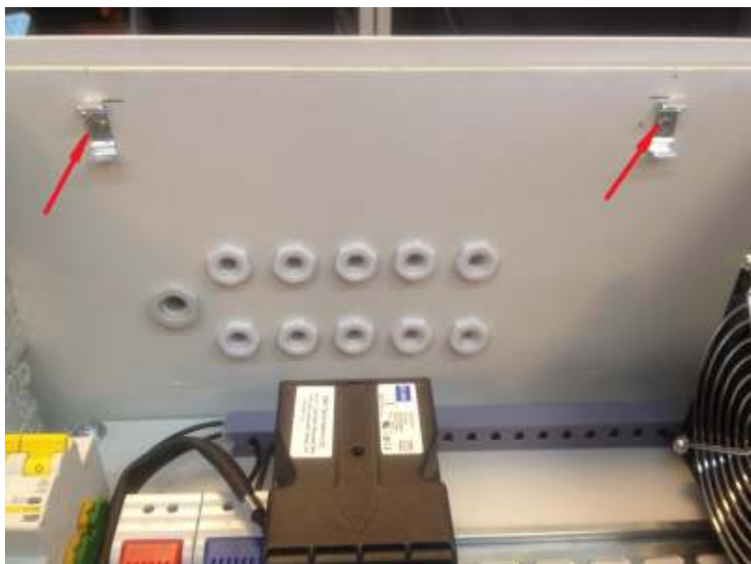
Рис.3.1.2-1 Установка пружинных креплений шкафа OSP.
