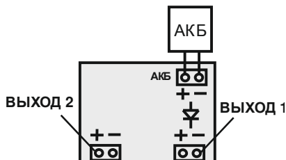
Рисунок 2 – Схема использования изделия в качестве зарядного устройства для АКБ
