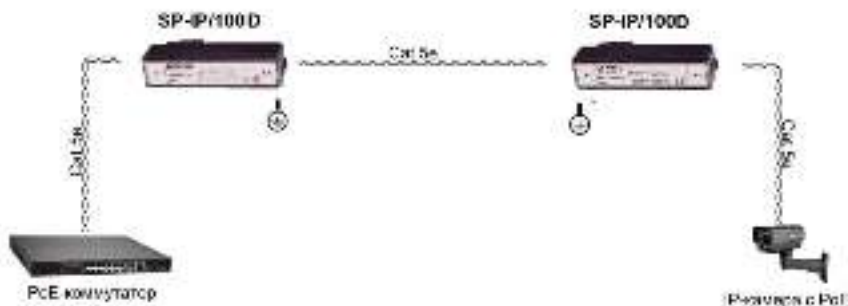
Рис. 10 Схема подключения SP-IP/100(ver.2) , SP-IP/100D , на примере SP-IP/100D .
