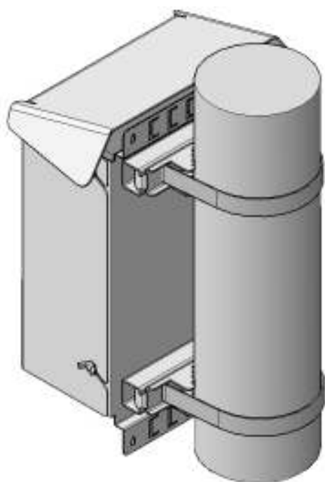
Рис. 2 Монтаж на круглую опору
