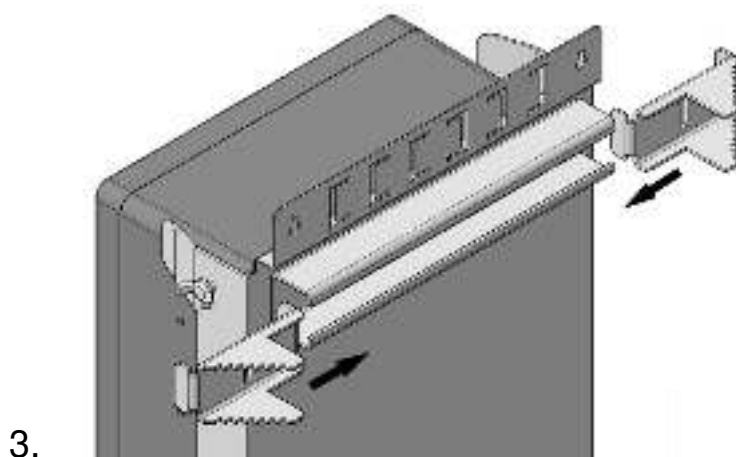
Рис. 1 Установка ККС-Hot на корпус коммутатора.
