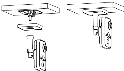
Рисунок 3-5 Установка камеры
