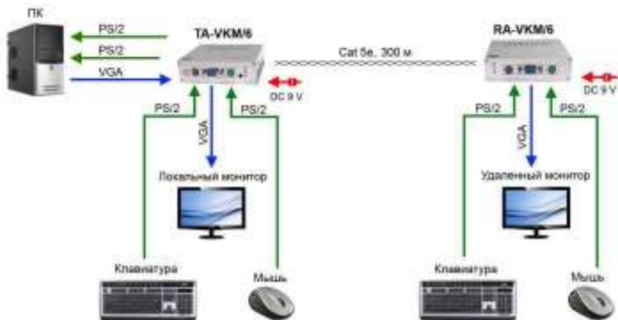
Рис. 5. Схема подключения TA-VKM/6+RA/VKM/6
