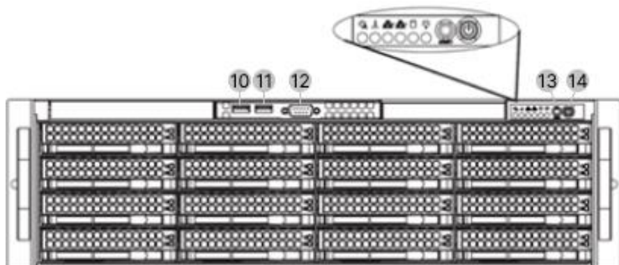
Рисунок 3. Передняя панель
