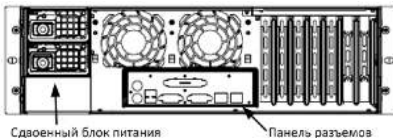
Рисунок 1. Задняя панель
