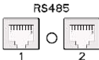
Назначение контактов разъема RJ-45 (порт RS485)
