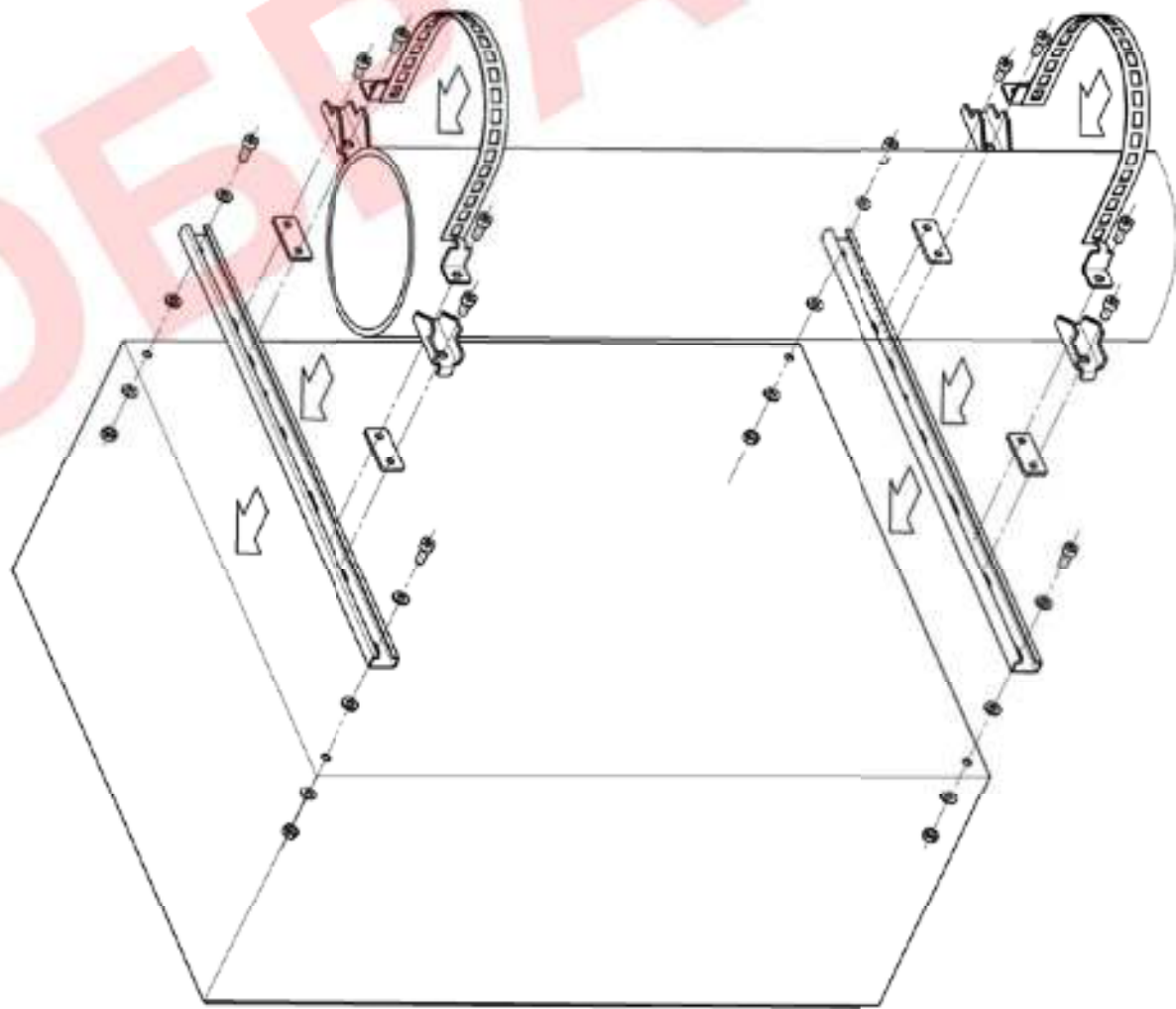
Рис.2 Установка на круглую опору
