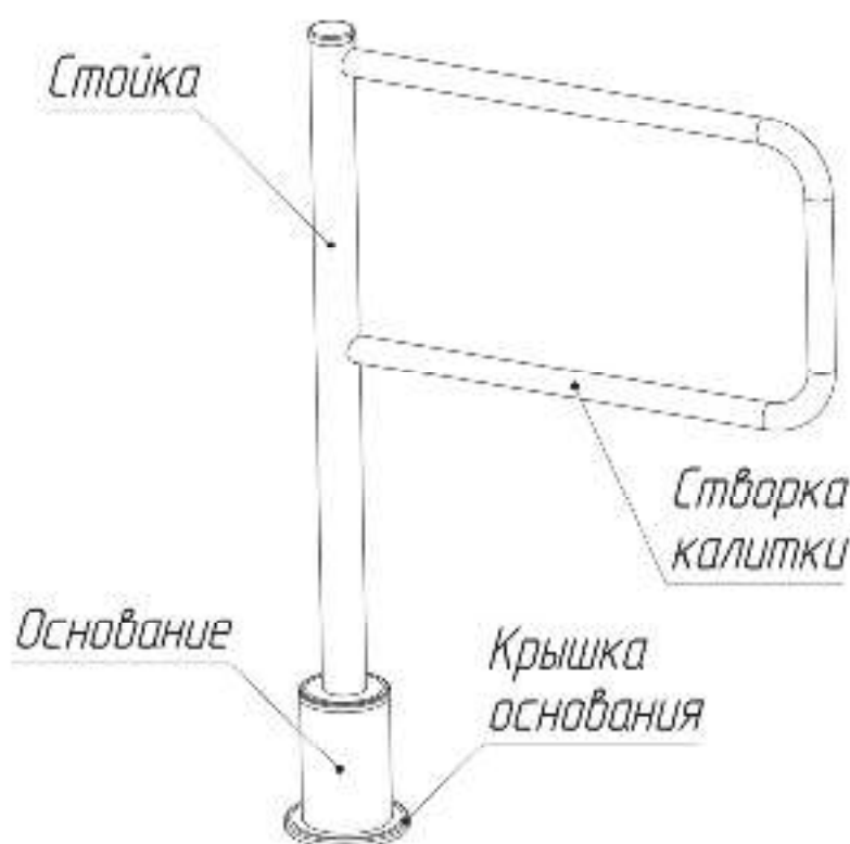
Рис. 1 . Общий вид
