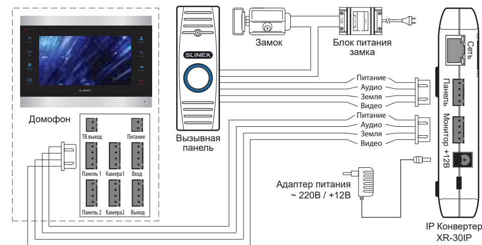
Схема 2. Подключение конвертера XR-30IP к сетевому интерфейсу посредством кабельного соединения.
