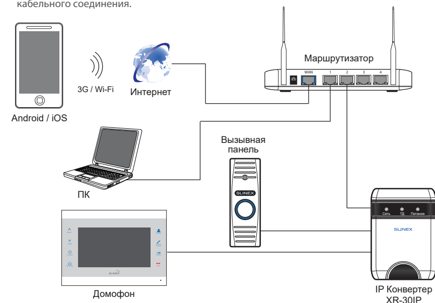
Схема 2. Подключение конвертера XR-30IP к сетевому интерфейсу посредством кабельного соединения.
